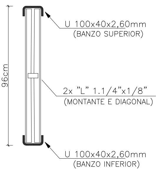
SEÇÃO TRANSVERSAL PILAR 01
