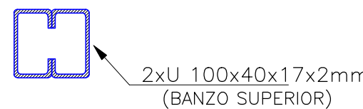
SEÇÃO TRANSVERSAL TUBO 02
