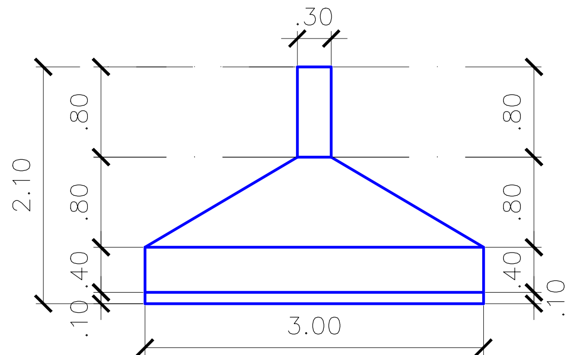
DETALHAMENTO 01
