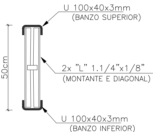
SEÇÃO TRANSVERSAL VIGA 02
