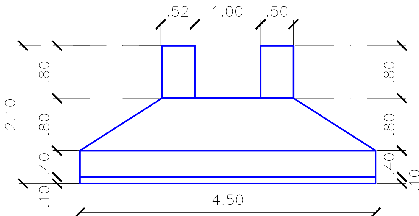
DETALHAMENTO 02
