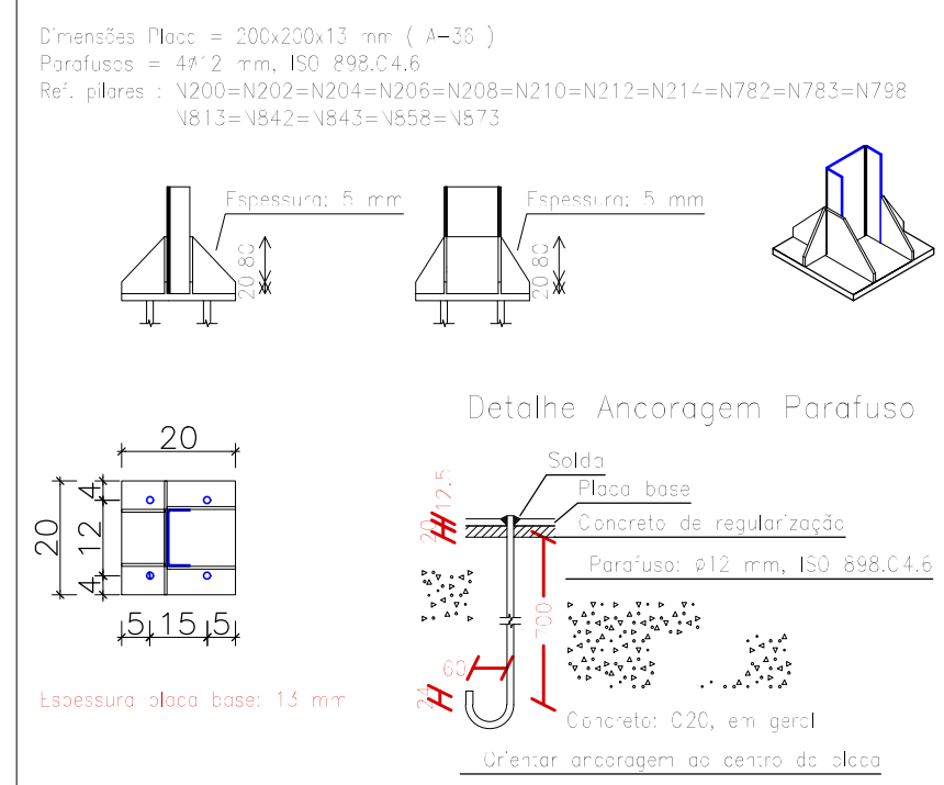
INSERT TIPO 1 – 16 UNIDADES
