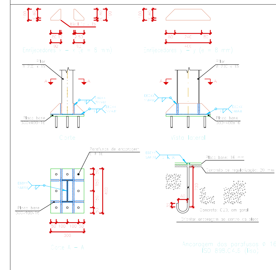
INSERT TIPO 2 – 08 UNIDADES
