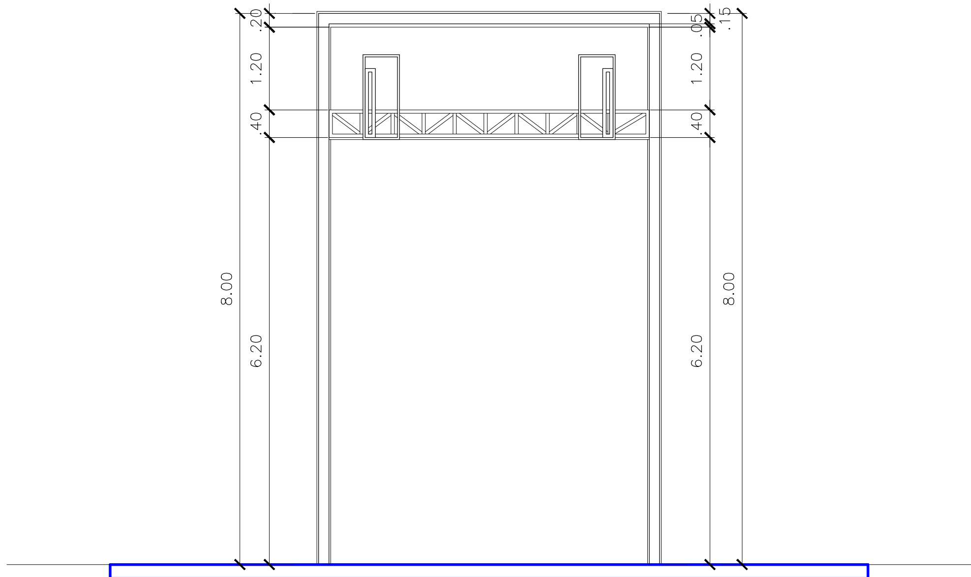
CORTE DD
