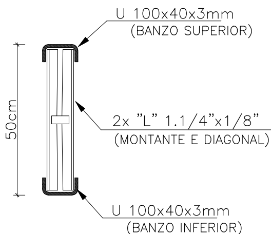
SEÇÃO TRANSVERSAL VIGA 01
