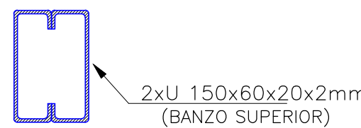
SEÇÃO TRANSVERSAL TUBO 01
