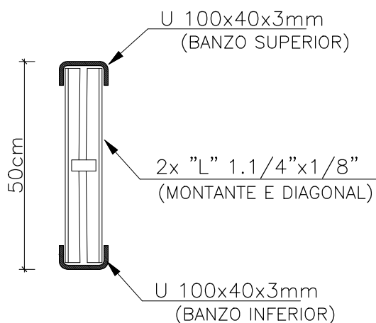
SEÇÃO TRANSVERSAL VIGA 03
