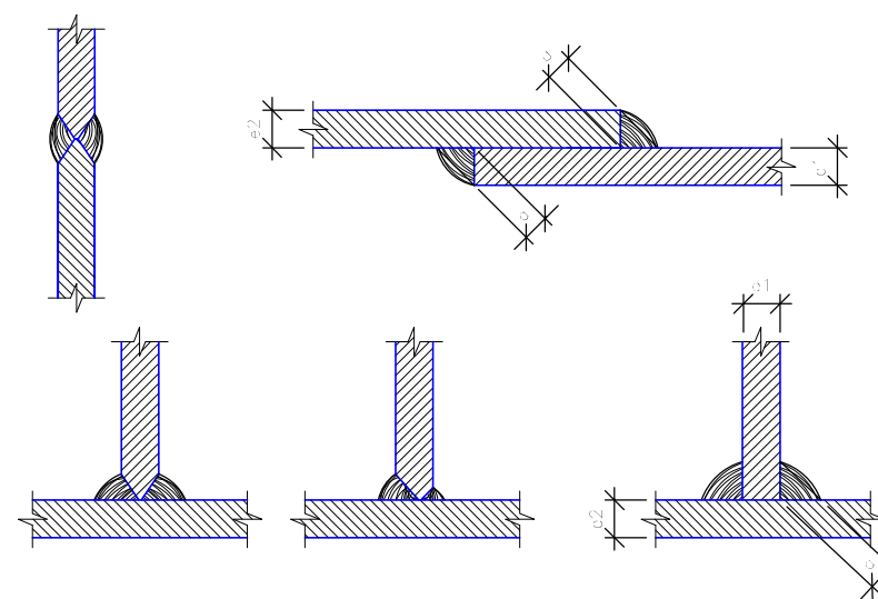
DET. TÍPICO TIPOS DE SOLDAS
