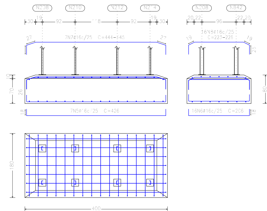
INSERT TIPO 1 – 16 UNIDADES
