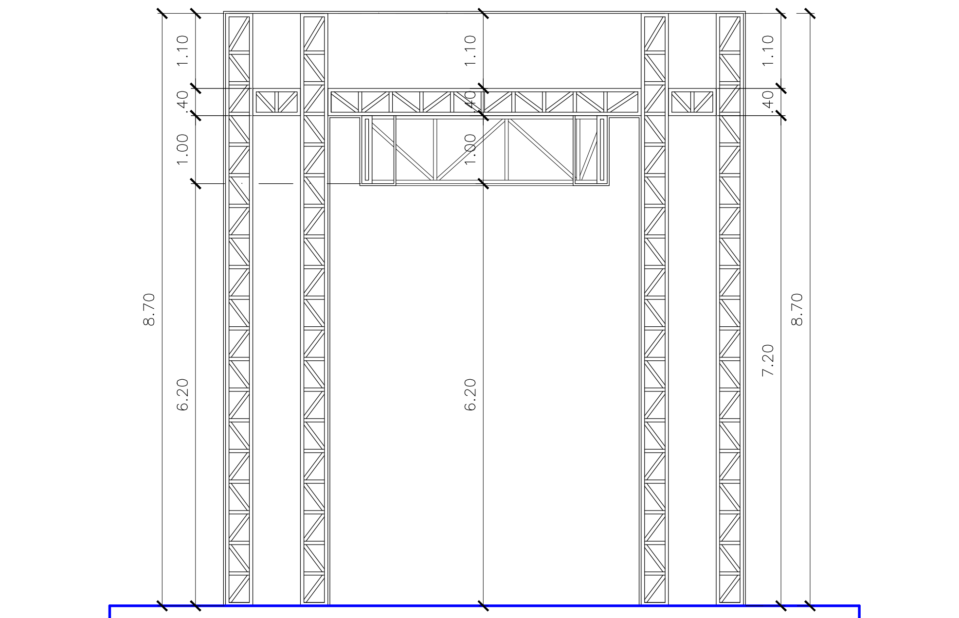
CORTE CC
