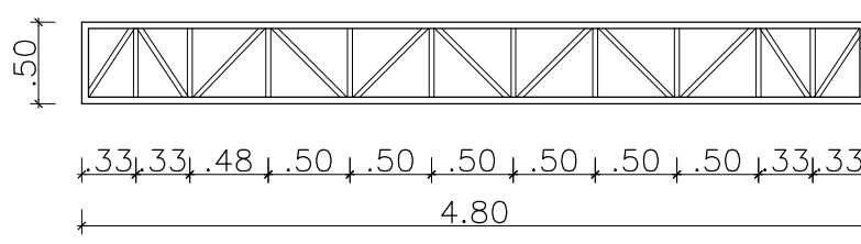
SEÇÃO TRANSVERSAL VIGA 03
