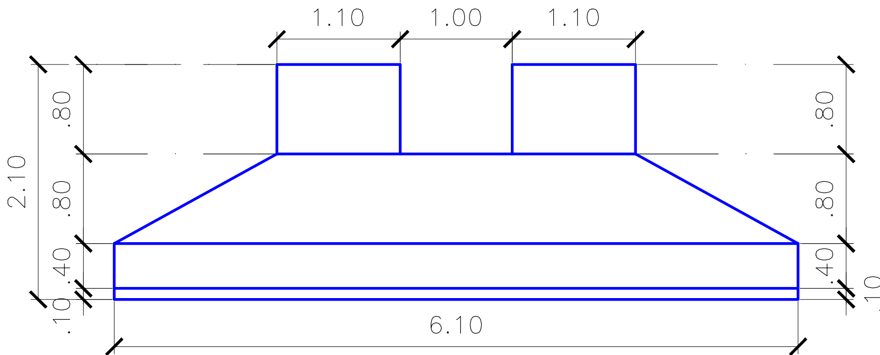
DETALHAMENTO 04
