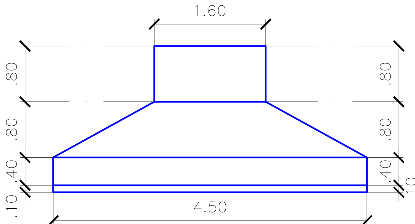
DETALHAMENTO 03
