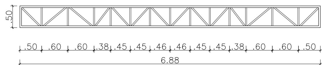
SEÇÃO TRANSVERSAL VIGA 01
