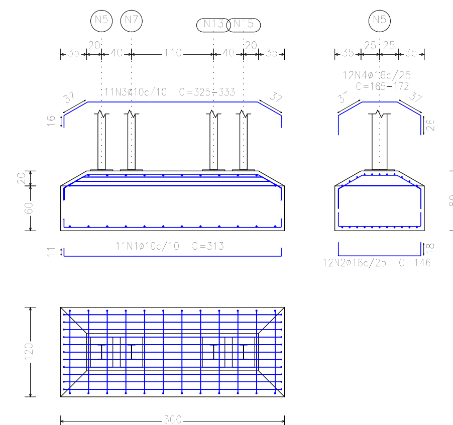
INSERT TIPO 2 – 08 UNIDADES
