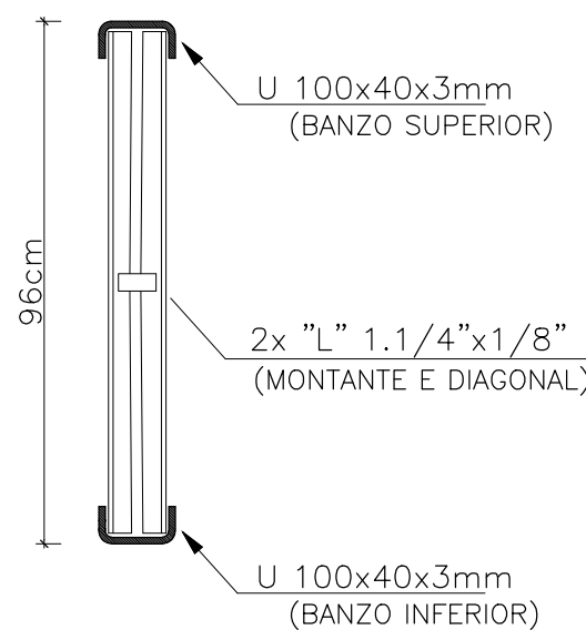
SEÇÃO TRANSVERSAL LONGARINA
