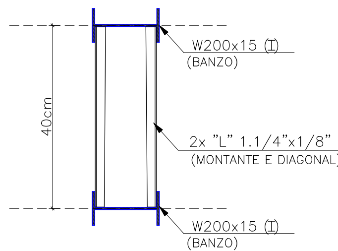
SEÇÃO TRANSVERSAL PILAR 02
